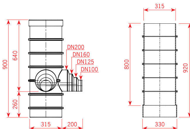
Šachta DN 315
